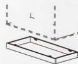
BASE GB 880 795W x 385D x 85H
